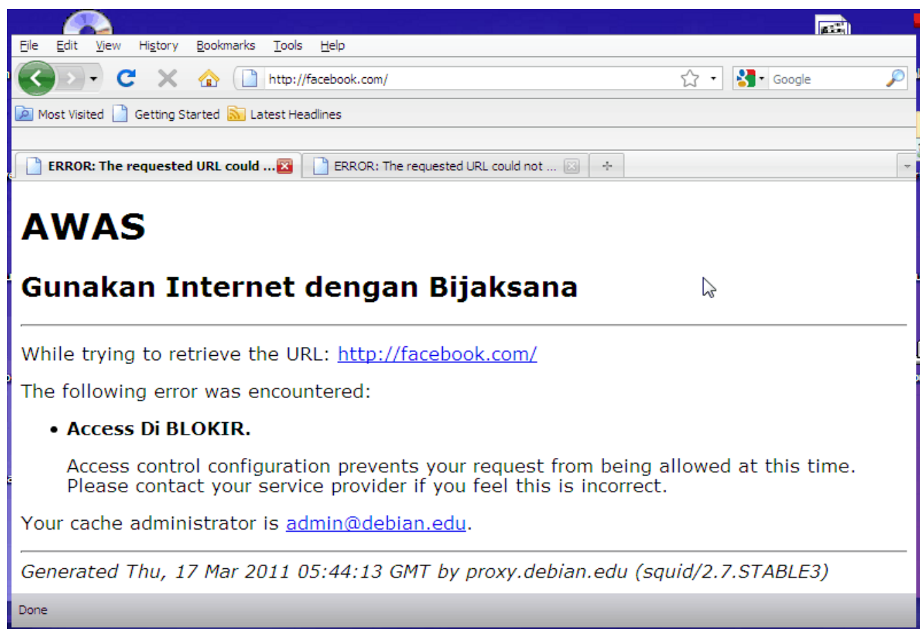
Gambar 23. Laman Blokir
